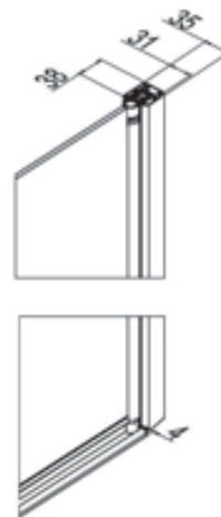
Paroi de douche d'angle, deux panneaux avec ouverture pivotante vers l'intérieur et l'extérieur. Hoekinstap met twee panelen, openzwaaiende panelen naar binnen en naar buiten.
