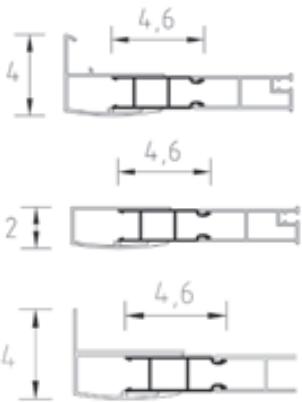
Profilé de compensation en option - Optionele compensatie profiel
