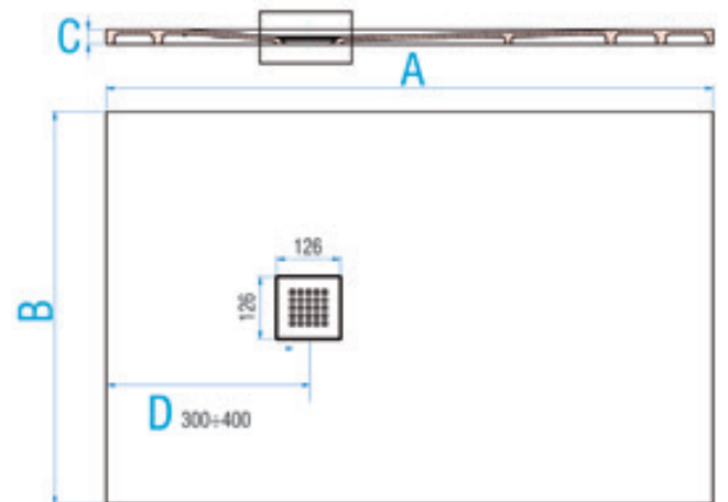
STONEFIT receveur encastré au niveau du sol STONEFIT inbouw, gelijk met de vloer ingewerkt
