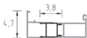
Profilé de compensation en option - Optionele compensatie profiel
