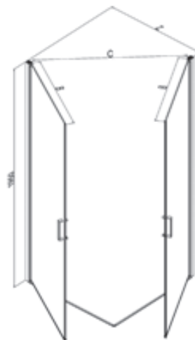
Paroi de douche d'angle, deux panneaux avec ouverture pivotante vers l'intérieur et l'extérieur. Hoekinstap met twee panelen, openzwaaiende panelen naar binnen en naar buiten.
