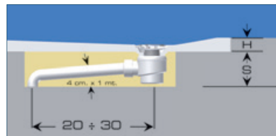
STONEFIT receveur encastré au niveau du sol STONEFIT inbouw, gelijk met de vloer ingewerkt
