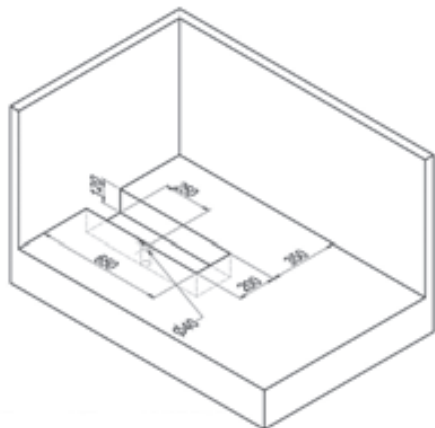
STONEFIT receveur posé sur le sol STONEFIT inbouw, vlak op de vloer geplaatst
