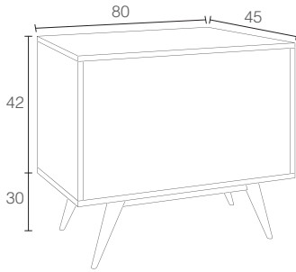
01 VINTAGE - Cajón / Tiroir / Drawer
